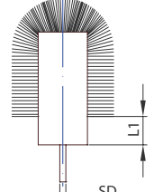
Rund mit Stift
