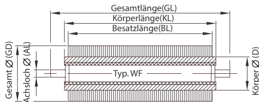
Typ Walzenbürste m. eingesetzten Achsenstummeln
