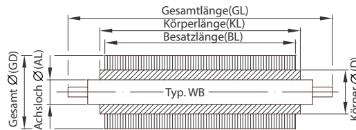
Typ Walzenbürste m. Welle Standard
